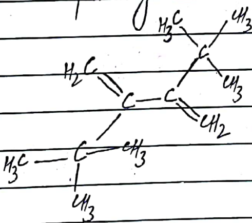
2,3-Di-tert-butyl-1,3-butadiene \lambda_{\text{max}} = 180\text{nm}
